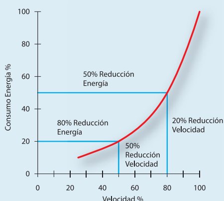
Consumo Ideal de Energía con Variación de Velocidad
