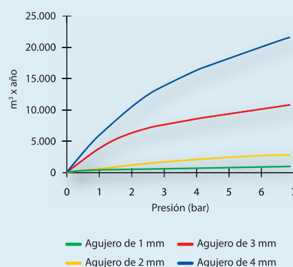
Pérdidas de Agua en un sistema de distribución
